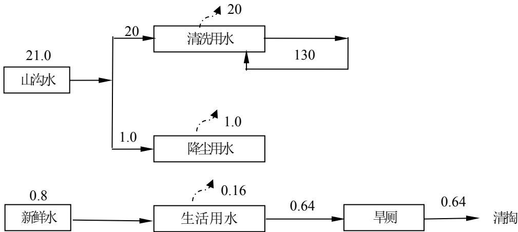
图 5-3 本项目水平衡图（单位：m³/d）
