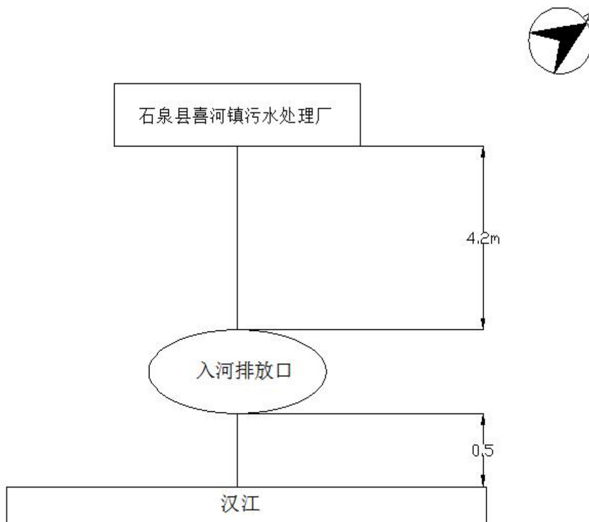
排污单位-排污管线-入河排污口-受纳水体排污走向图:
